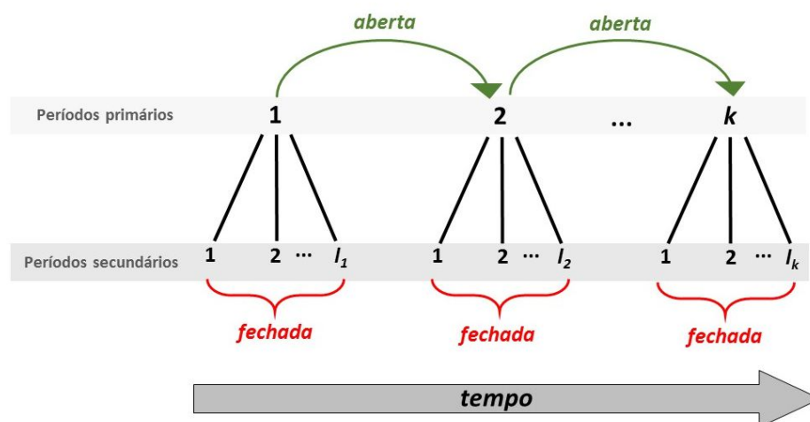
Figura 3.1 - Estrutura clássica referente ao desenho robusto de Pollock. Entre os k períodos primários a população é considerada aberta, ao passo que nos l_k períodos secundários o fechamento populacional é admitido.
